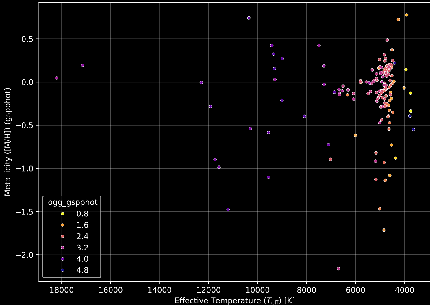
APOGEE DR17 Field: [068-04] Stellar Population Parameters (n= 168)
